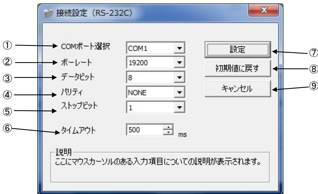
図 5-3 RS-232C 設定
