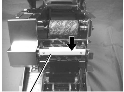
リボンピンチレバー
