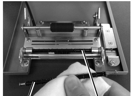
ハクリローラー① ハクリローラー②
