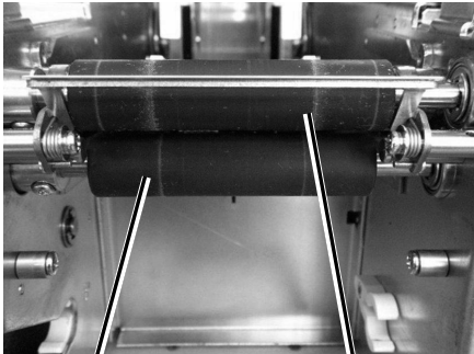
ハクリ搬送ローラー プラテンローラー
