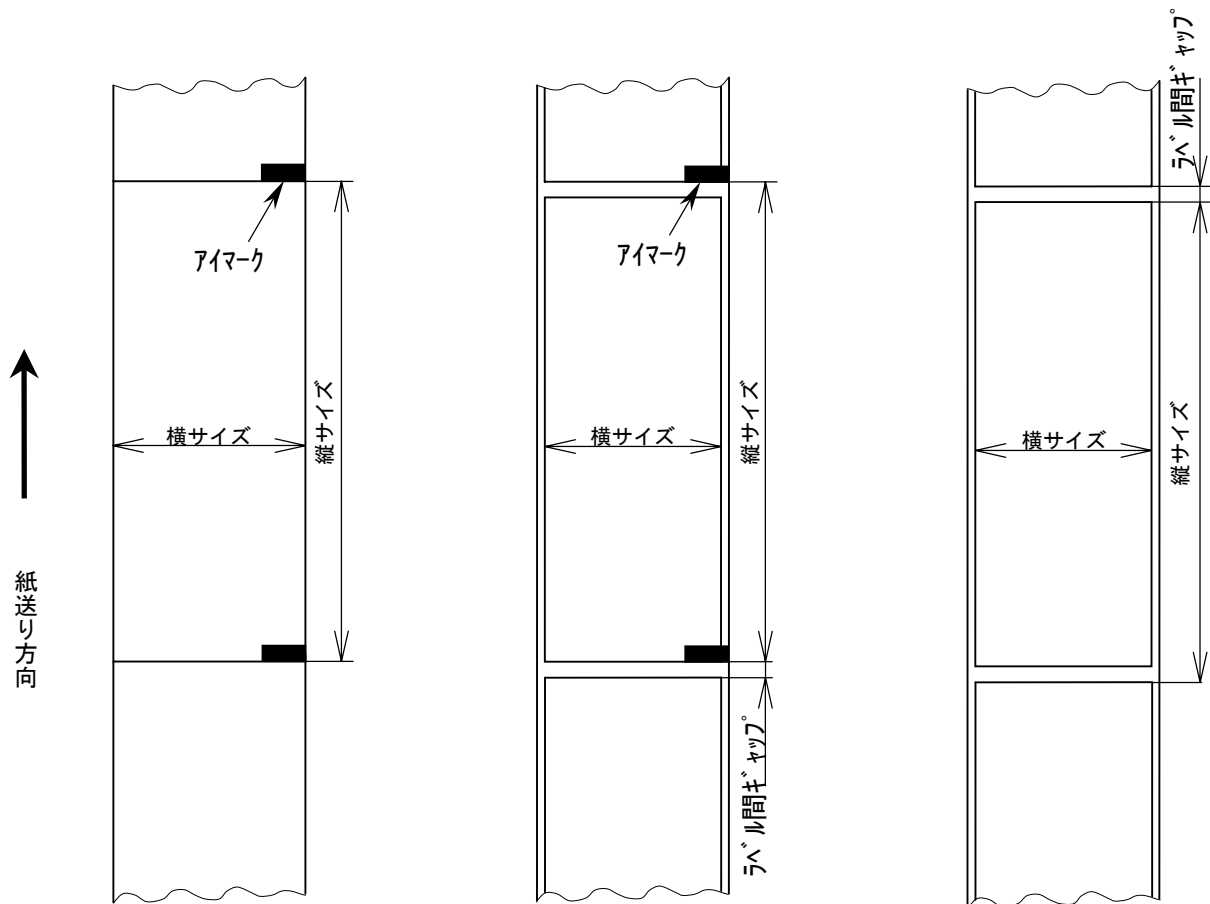
(a) のりなしタグ・裏アイマーク (b) のりつきラベル・裏アイマーク (c) のりつきラベル・ギャップ
