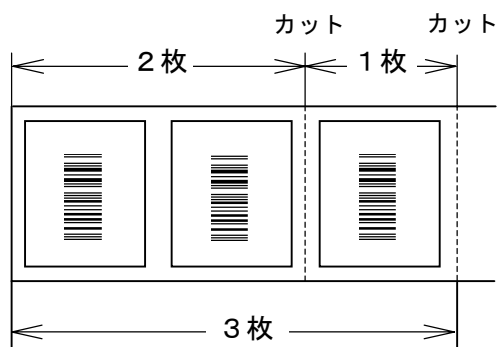
図 9-2. 「CT」コマンドによるカット動作
